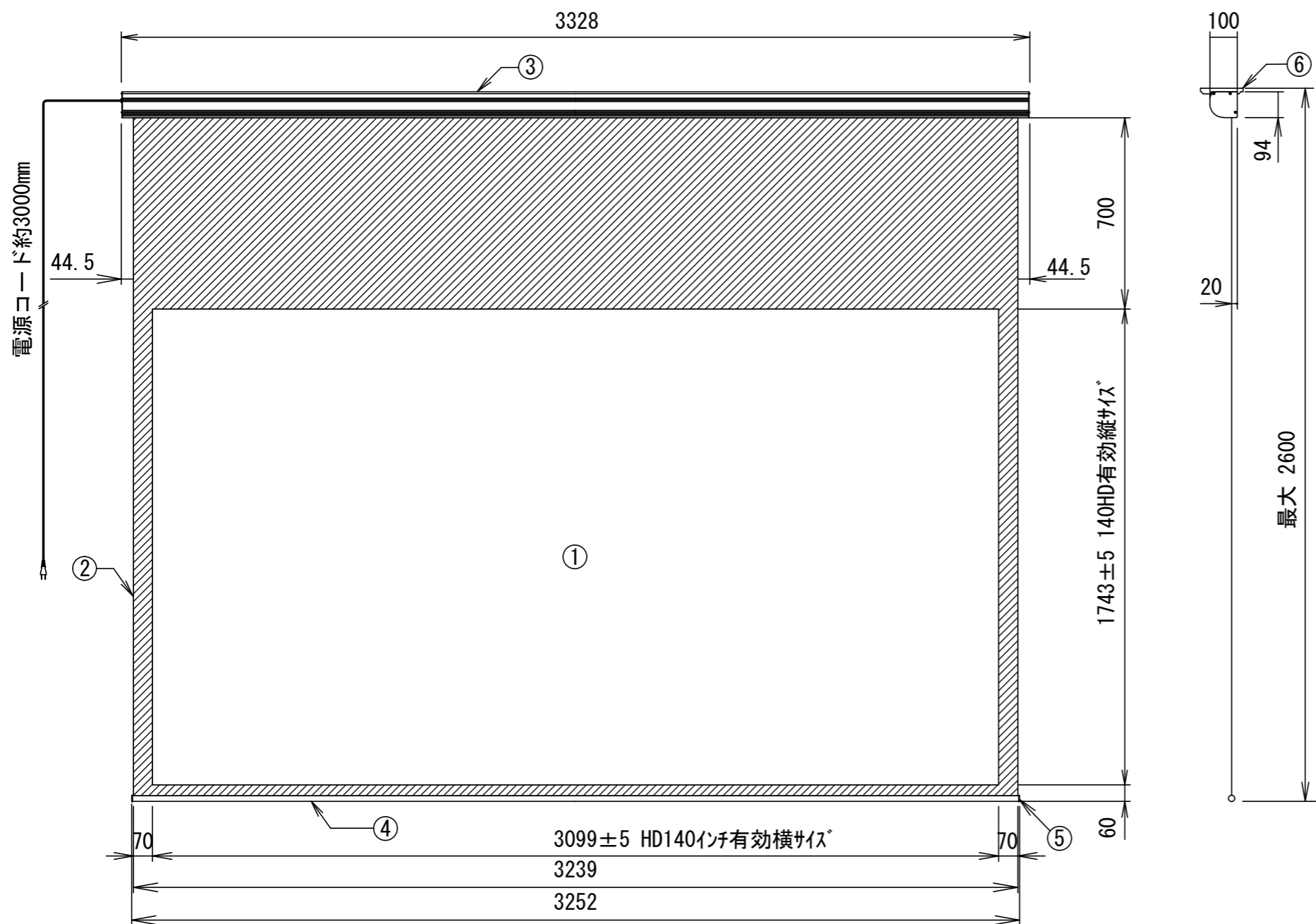
正面図
