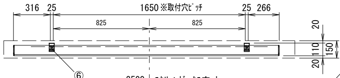
平面図
