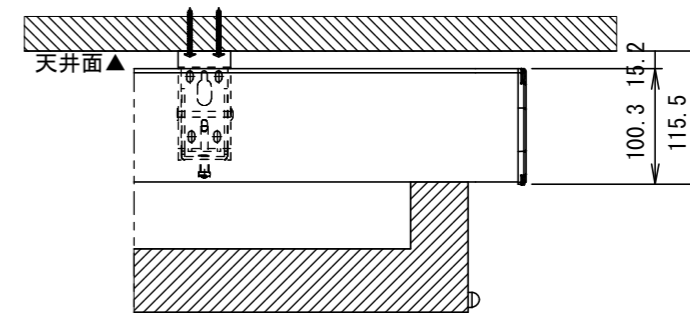
正面図
