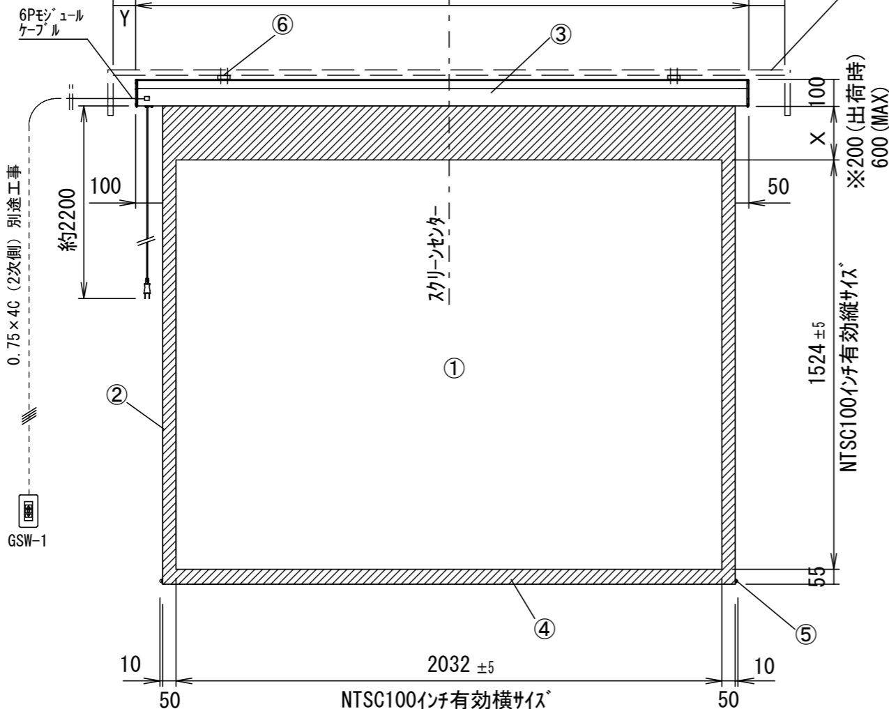
正面図
