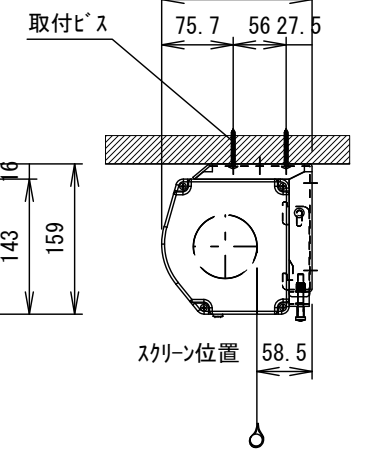
右側面図
