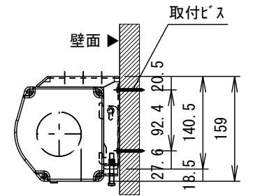
右側面図
