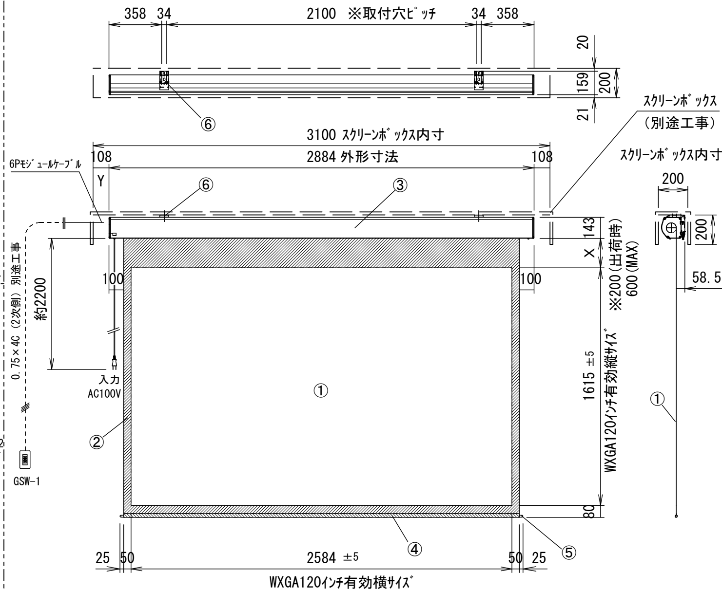
正面図
