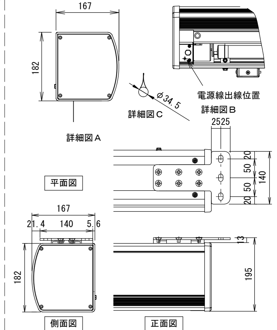
詳細図 S=1/6
