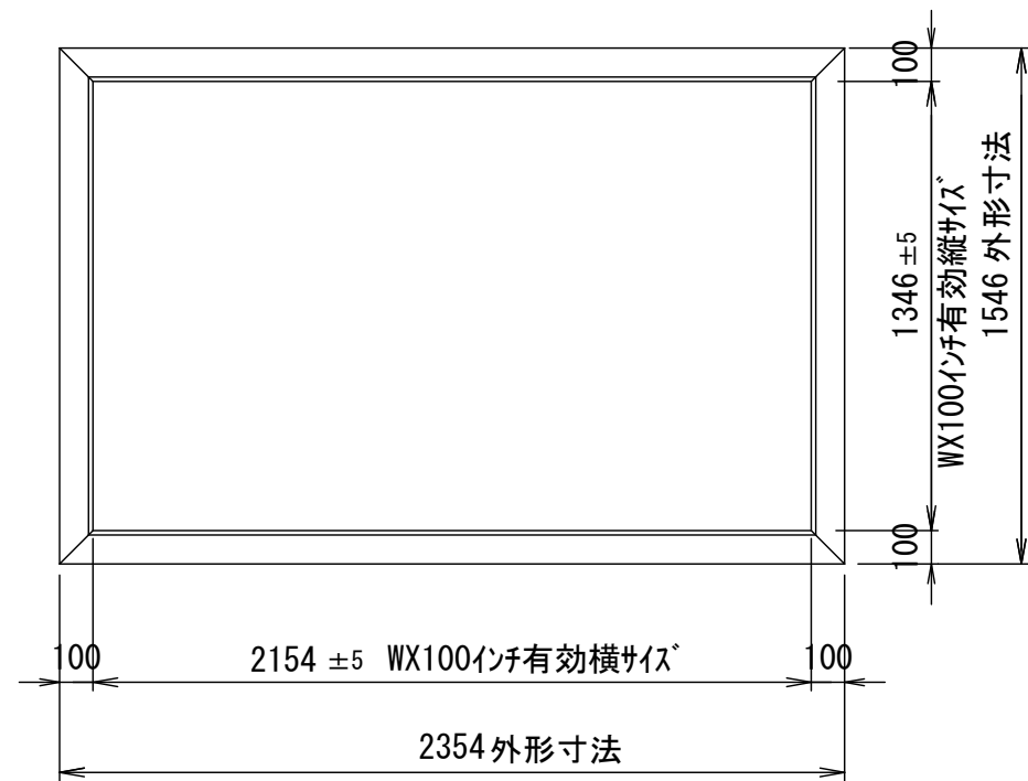
正面図
