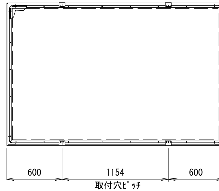
背面図
