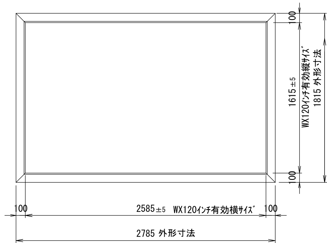
正面図
