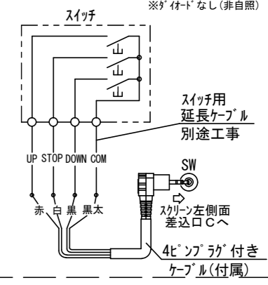
詳細図S=1/6
