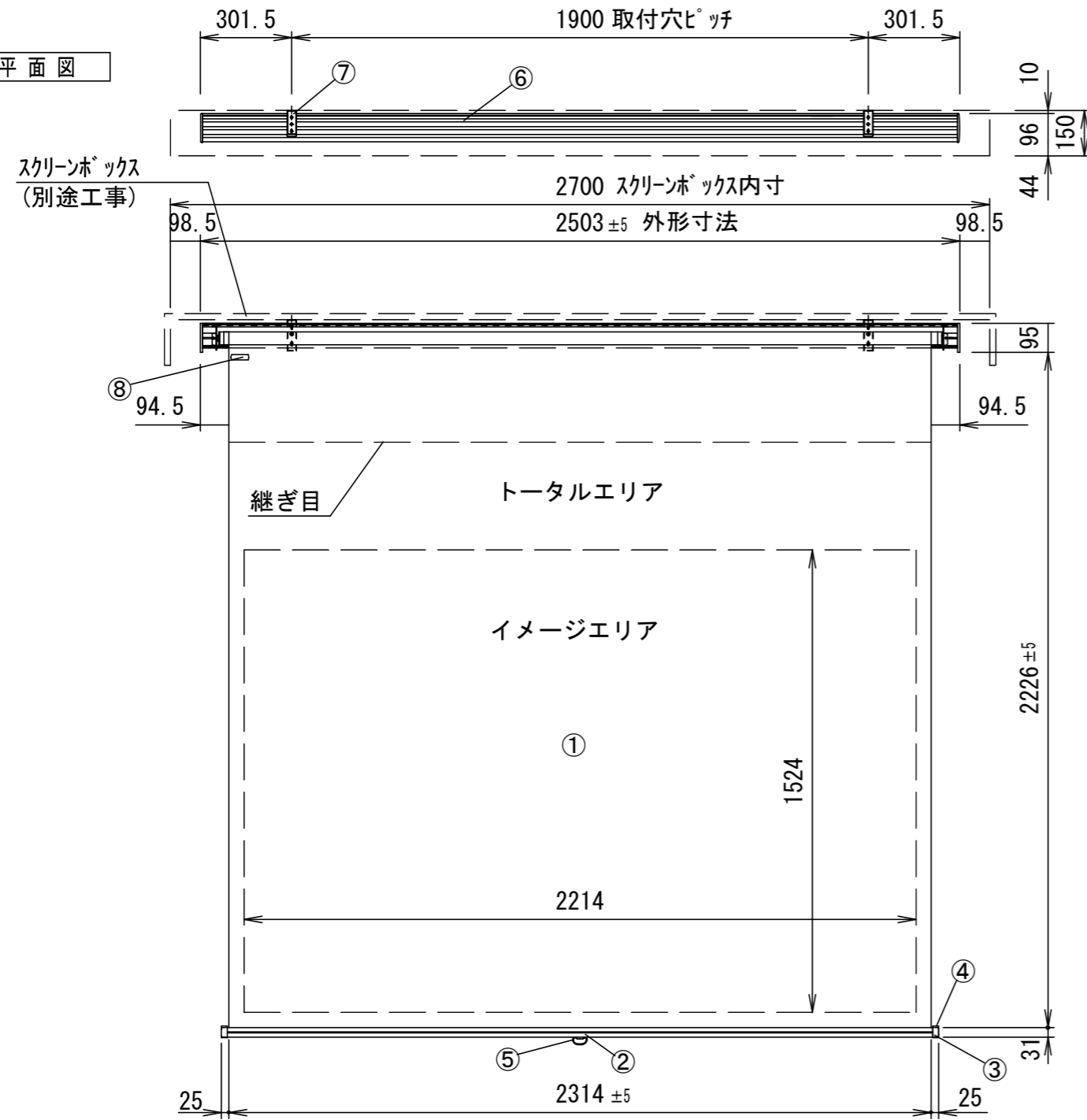
正面図
