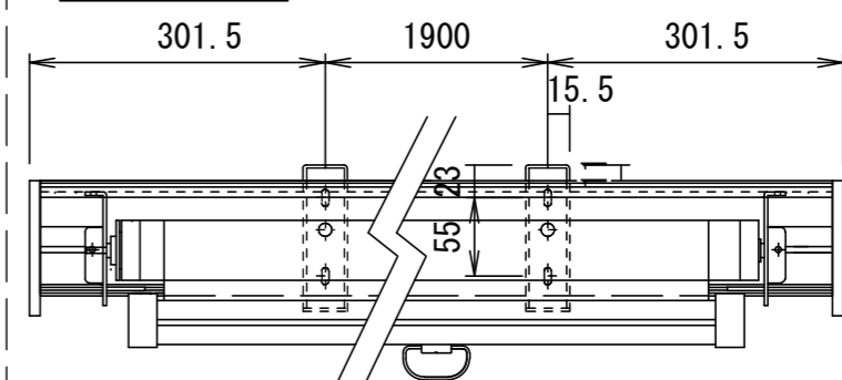
壁面取付時
