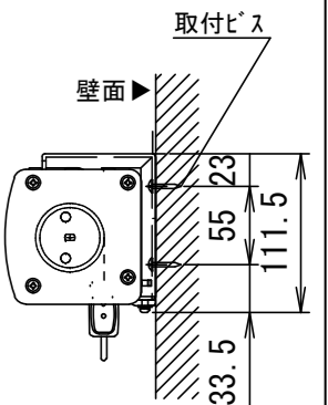
右側面図
