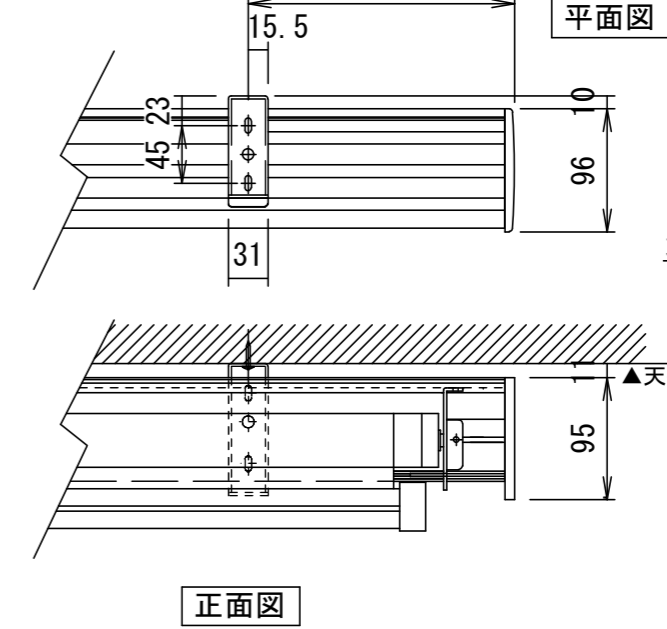
壁面取付時
