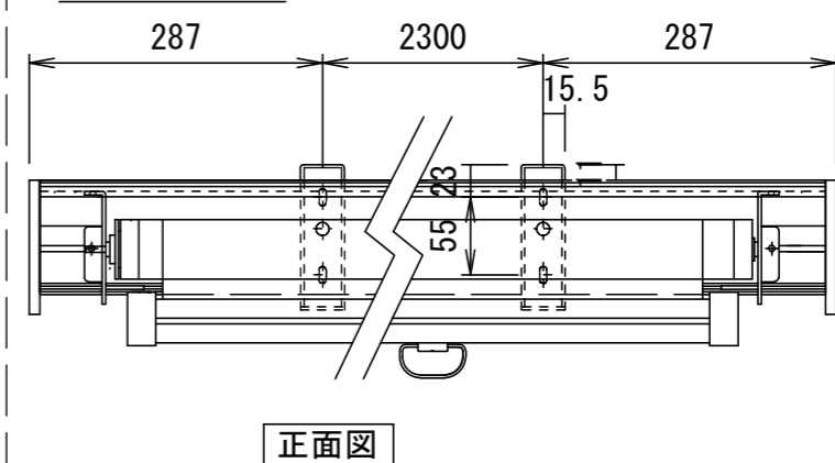
壁面取付時
