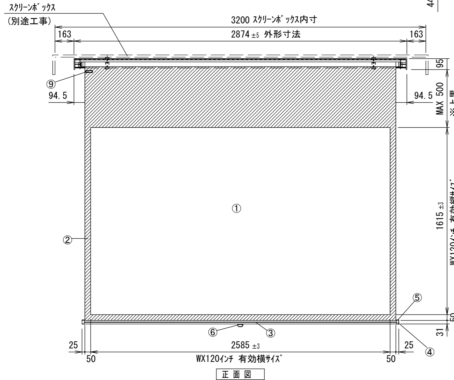
各部名称
