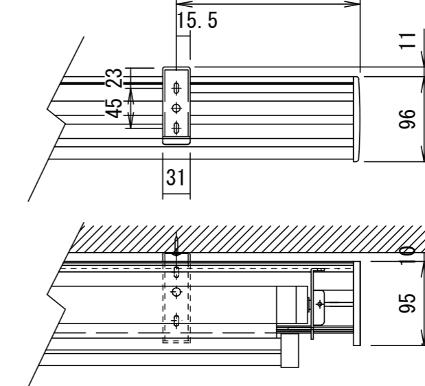
天井取付時
