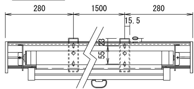
壁面取付時
