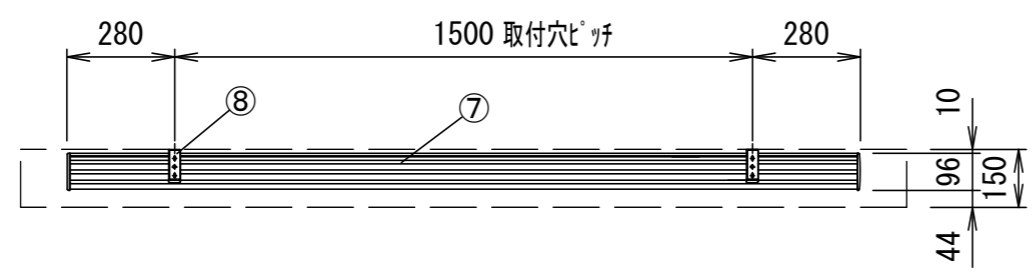
平面図
