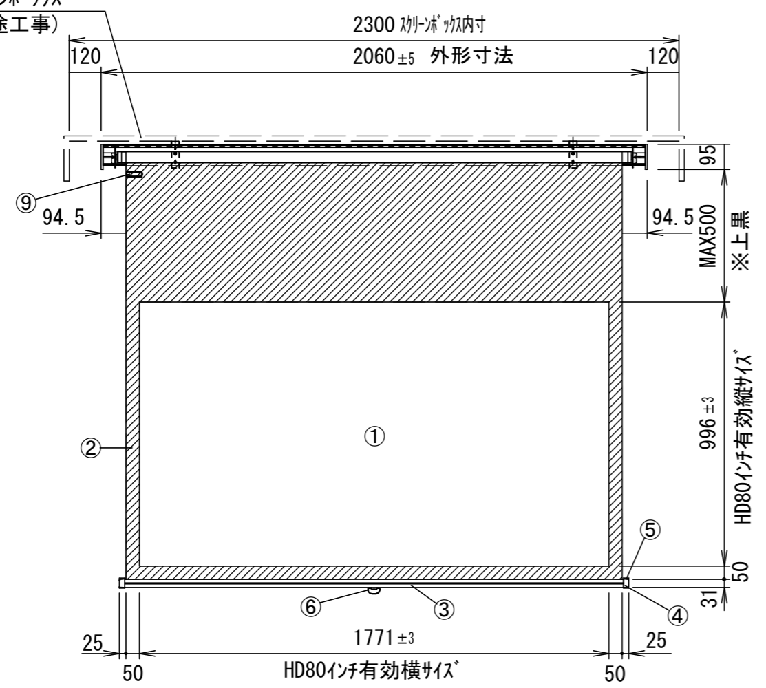
正面図
