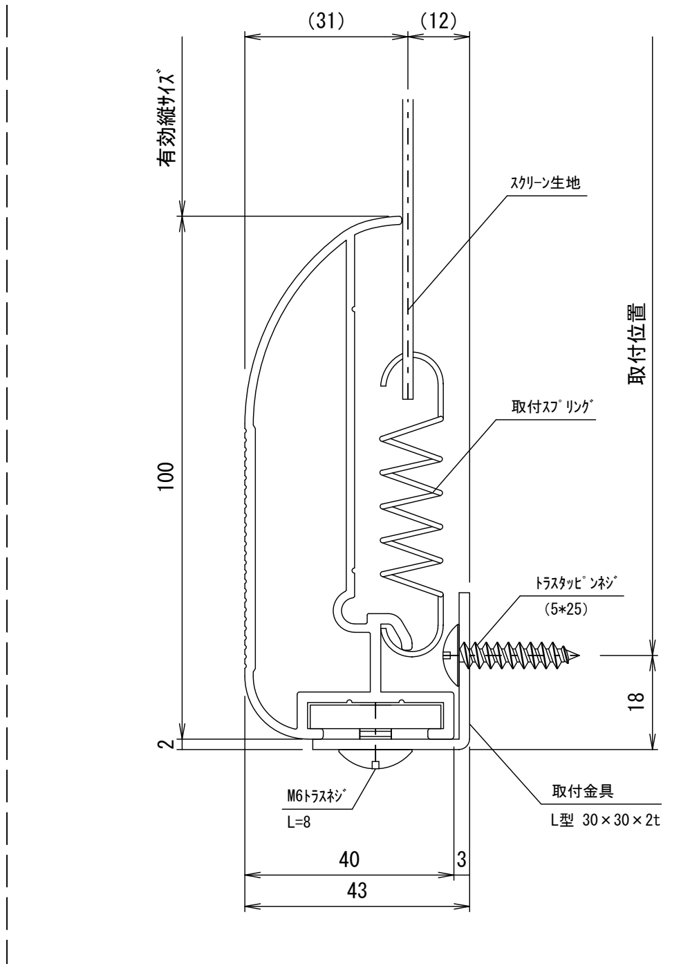
A 断面図 S = 1 / 1
