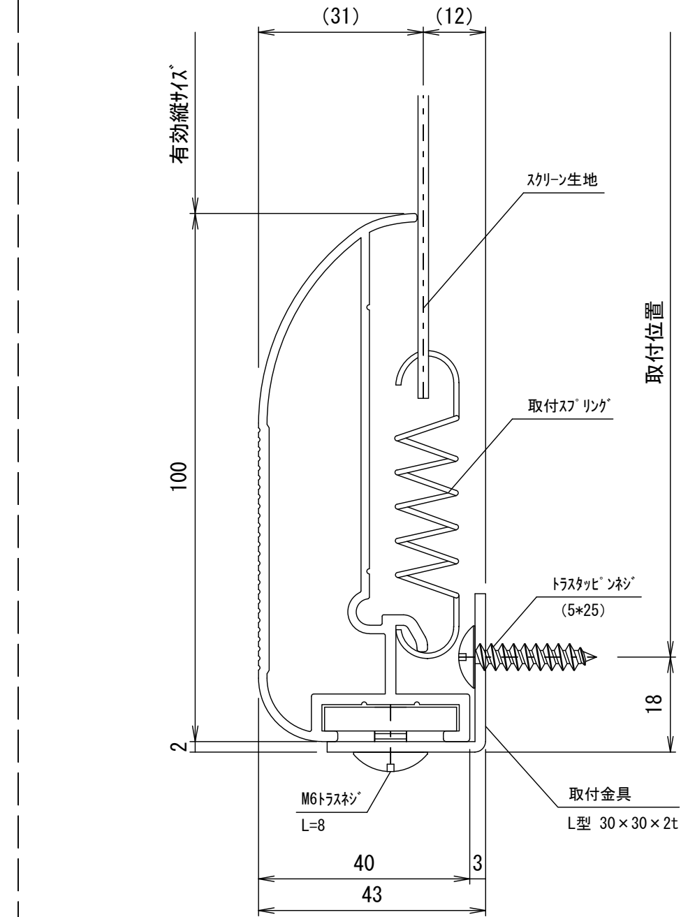
A 断面図 S = 1 / 1
