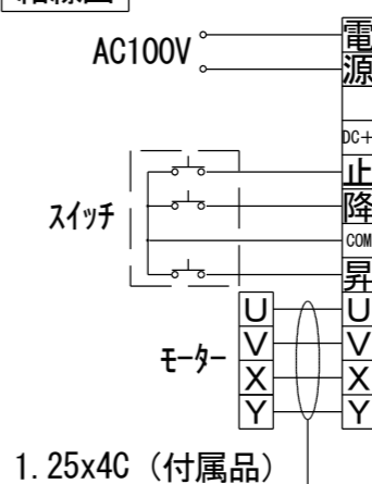
結線図
