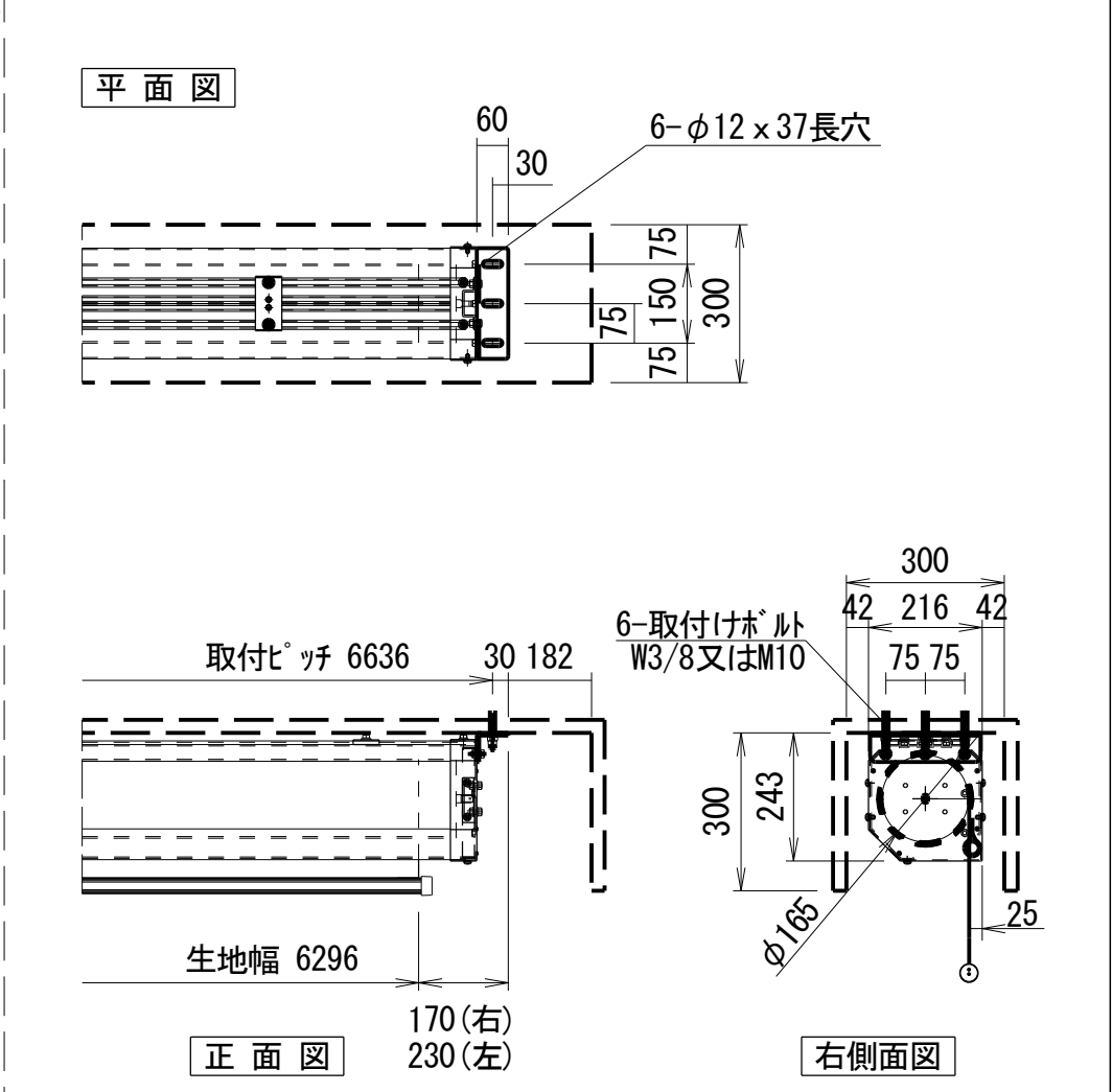
詳細図 1/15
