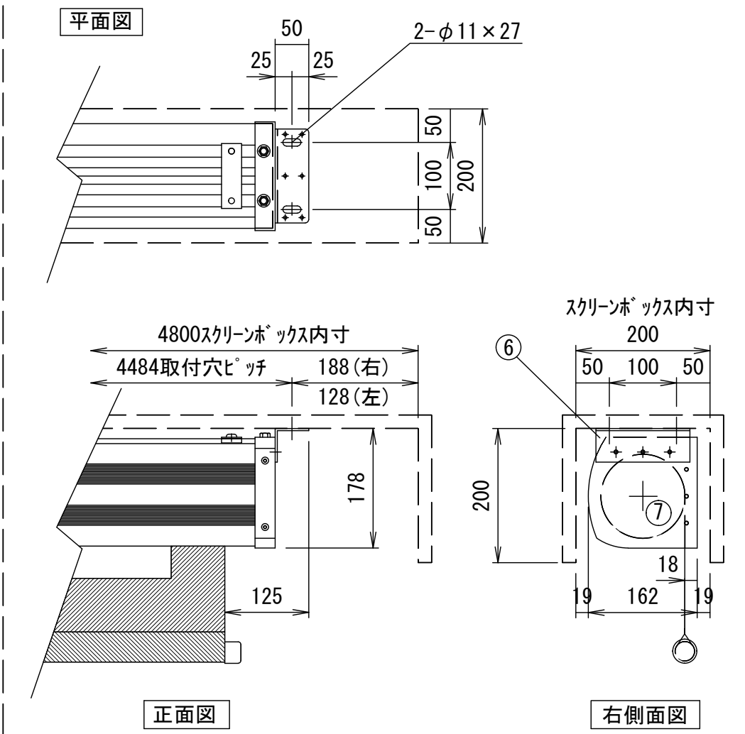
詳細図S=1/8
