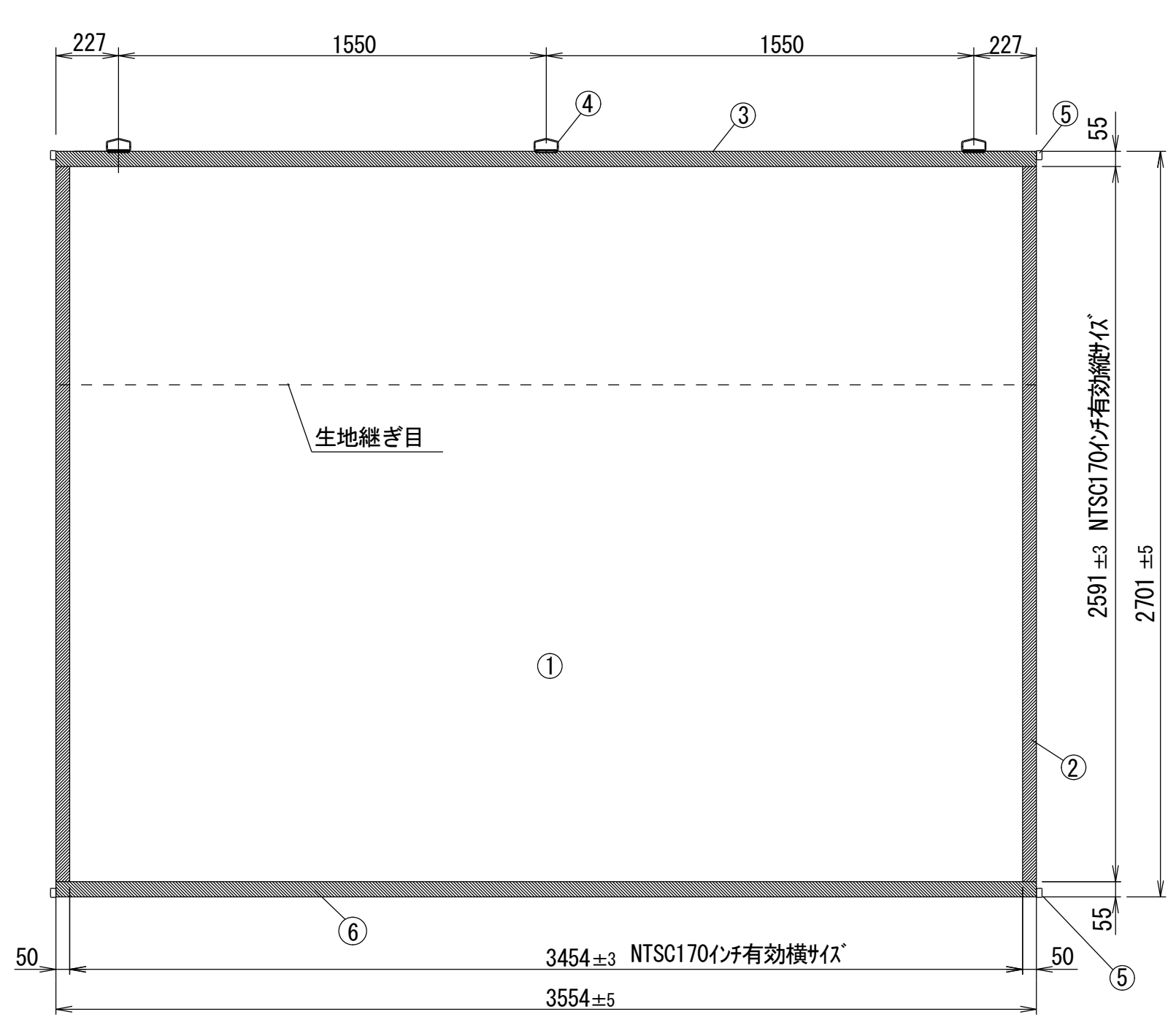
正面図
