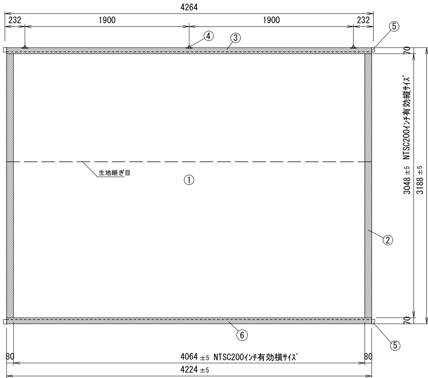
正面図
