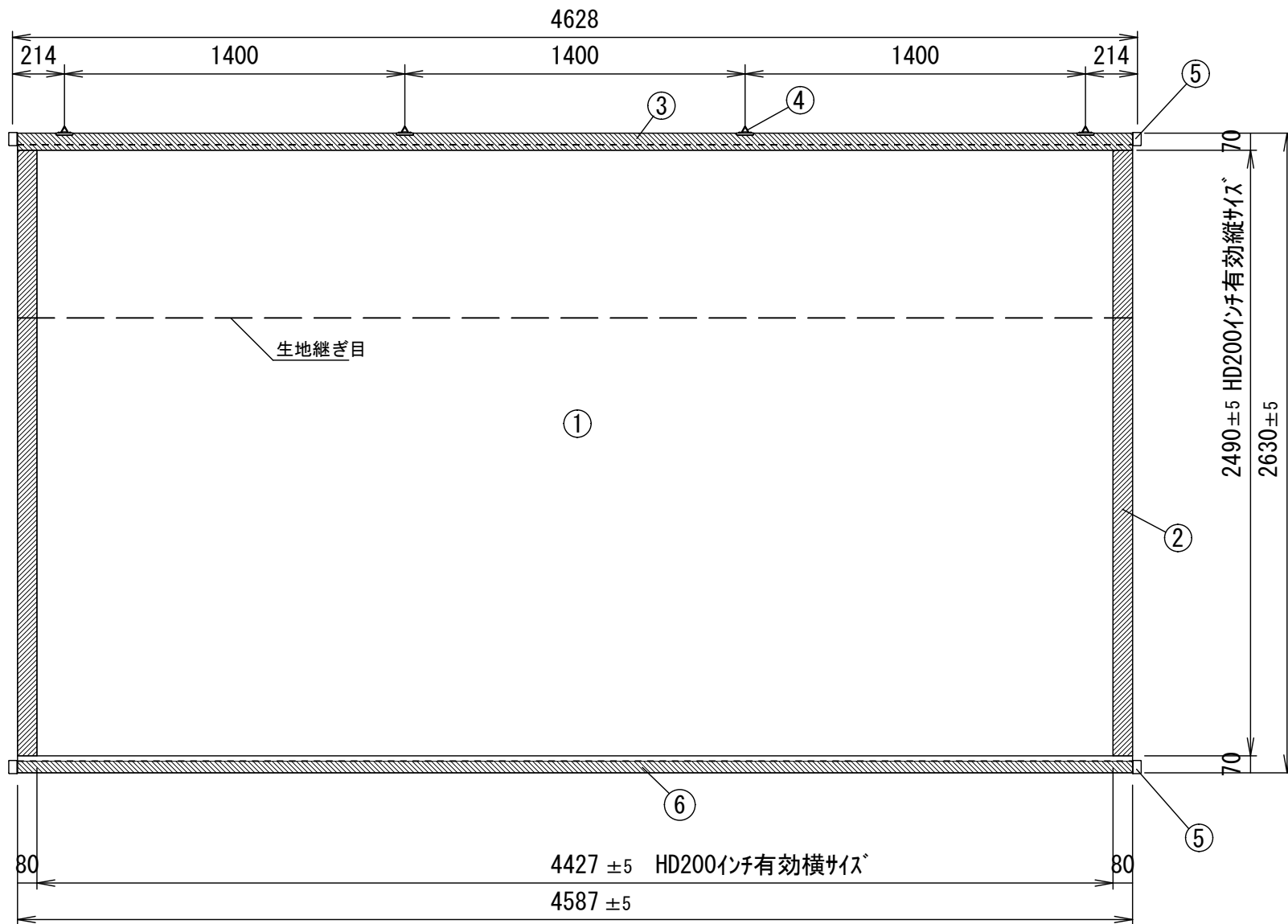
正面図
