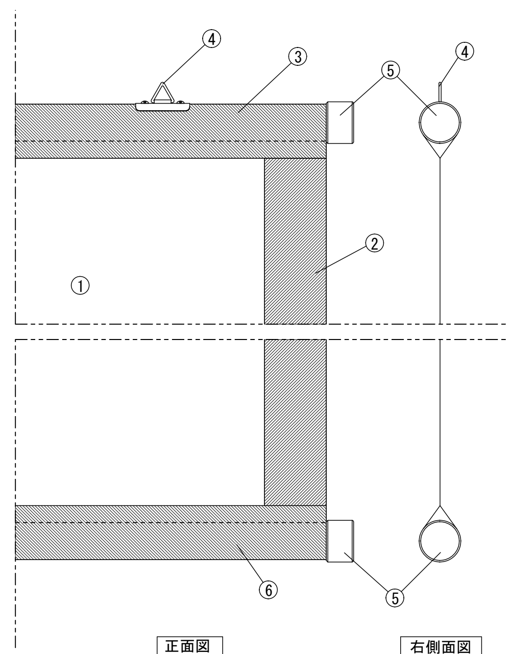
詳細図S=1/5
