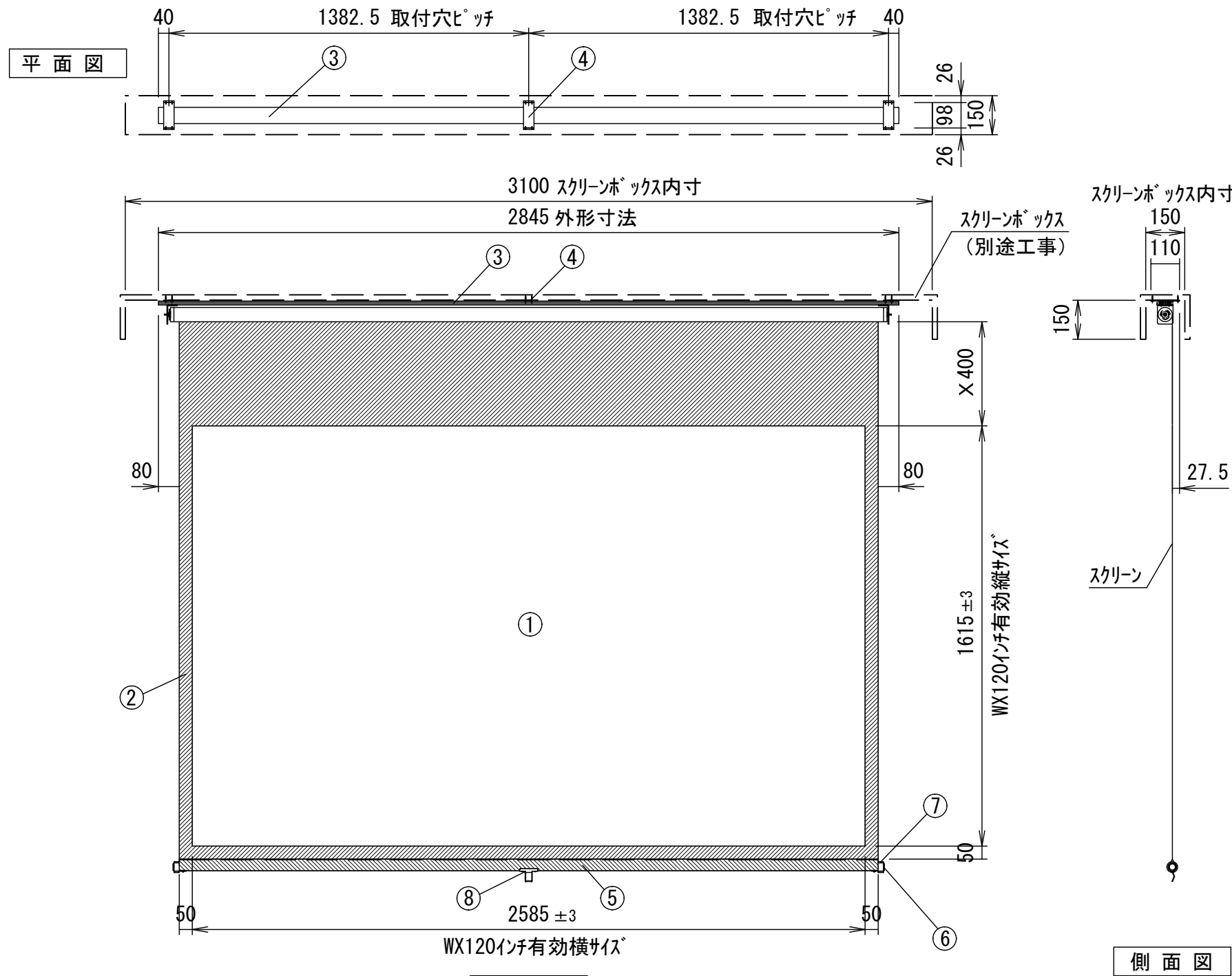
正面図
