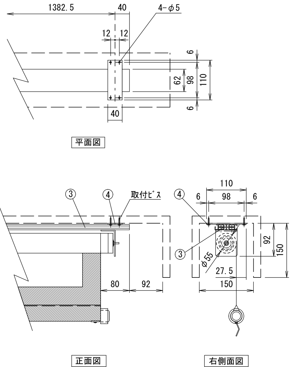
詳細図S=1/6
