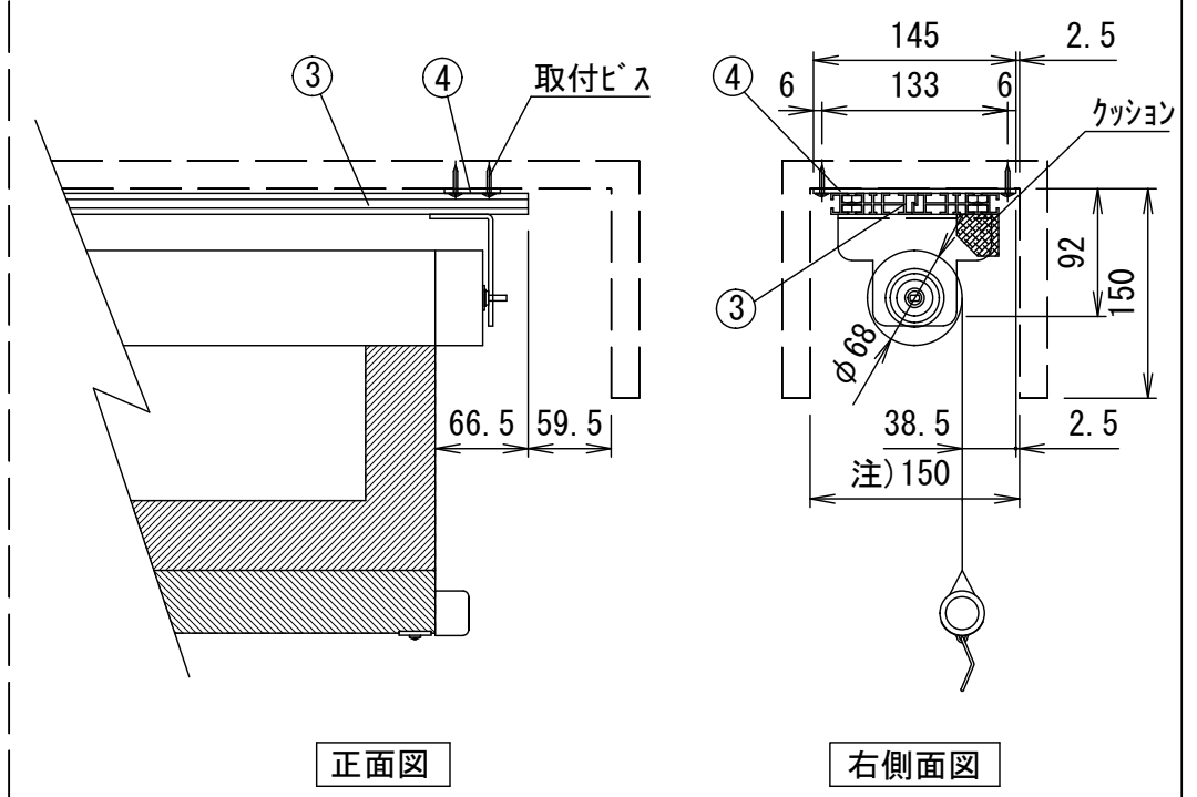
詳細図S=1/6
