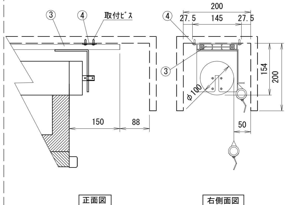
詳細図S=1/6
