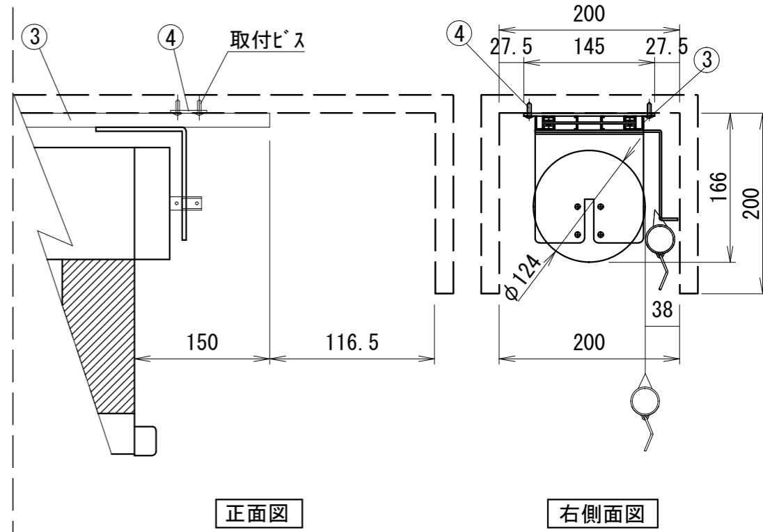
詳細図S=1/6
