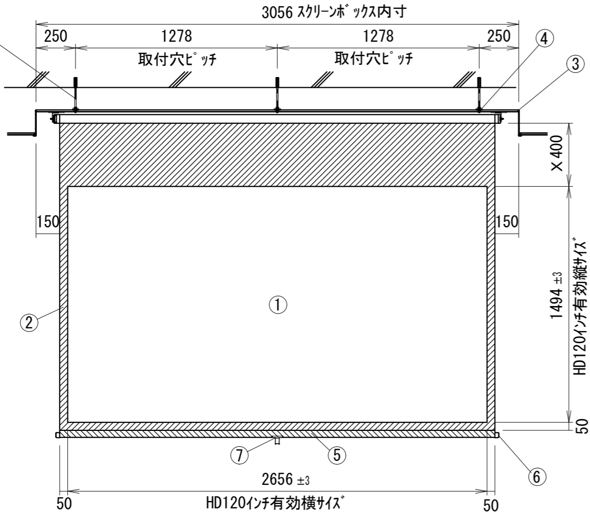
正面図
