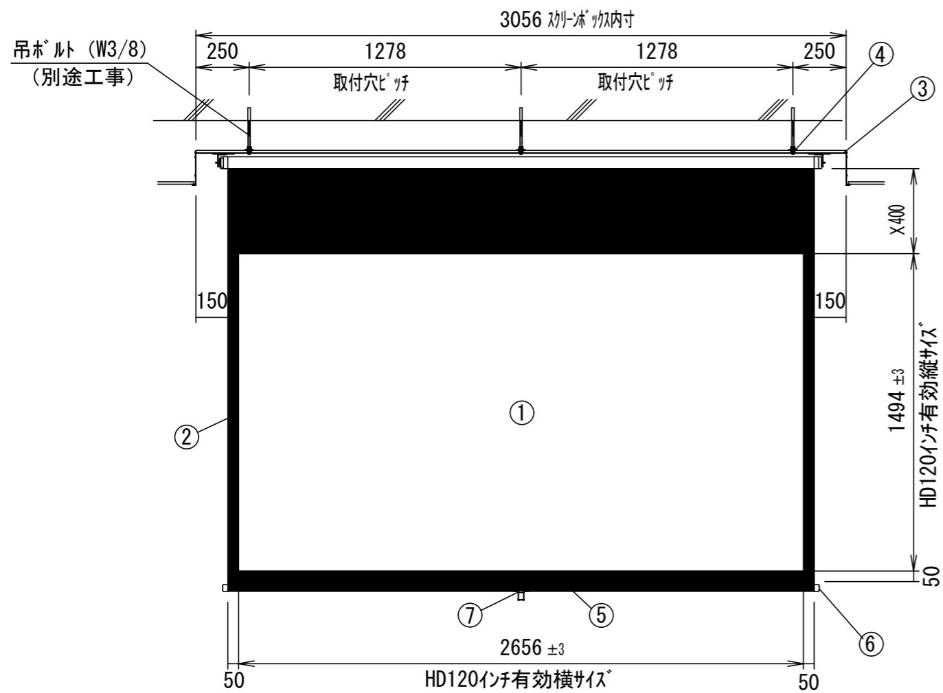
正面図
