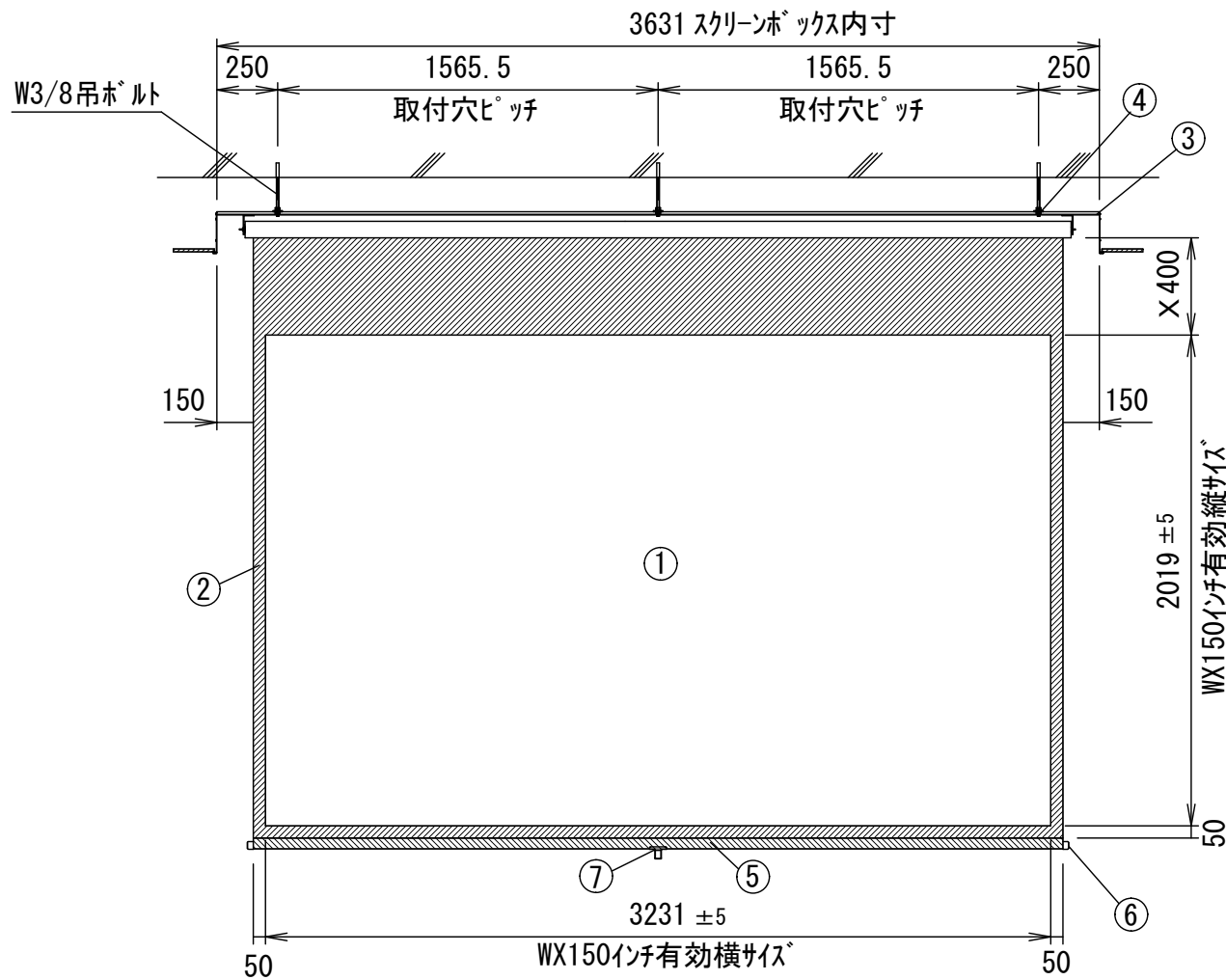
正面図
