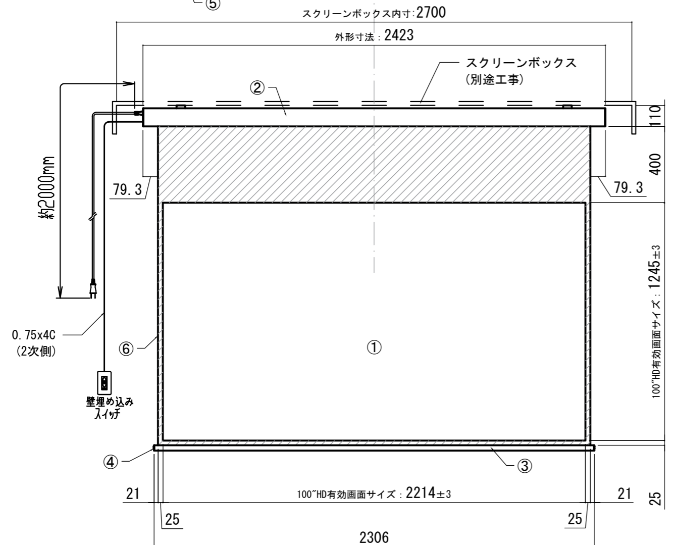
正面図
