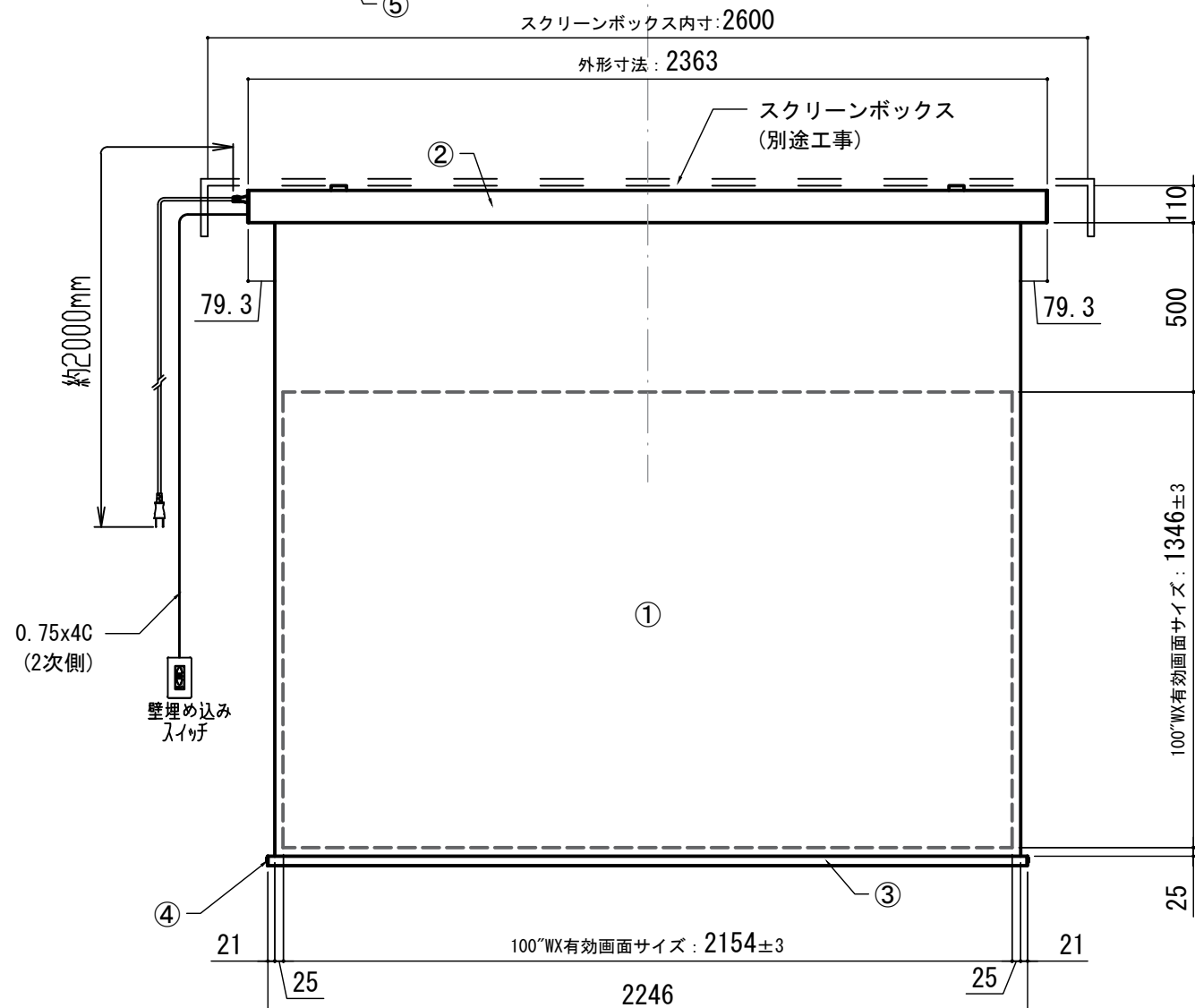
正面図
