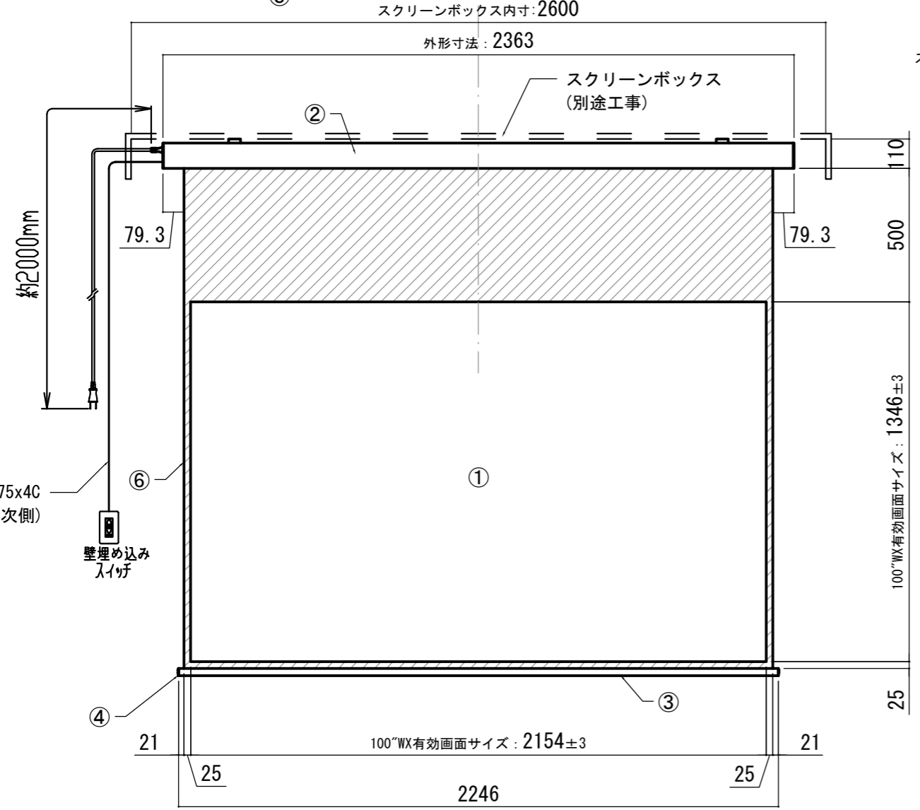
正面図
