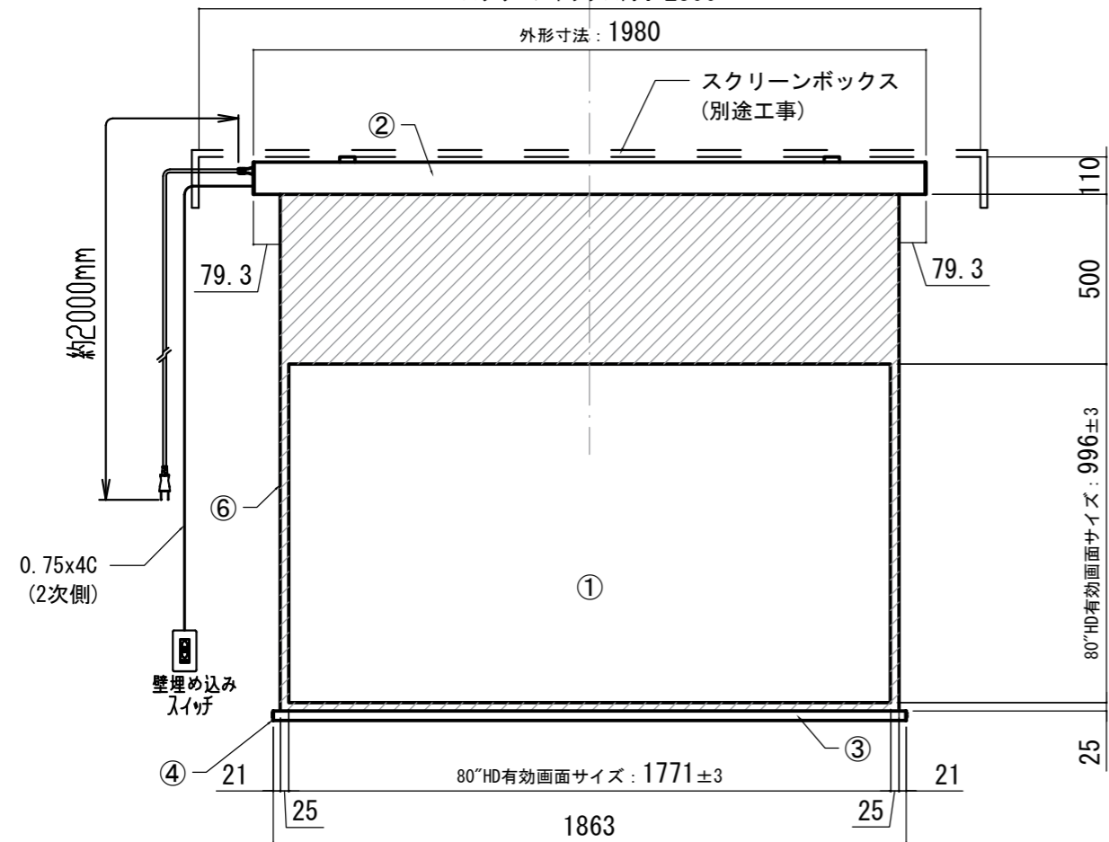
平面図
