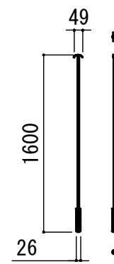
プルバー(引下げ棒) S=1:30
