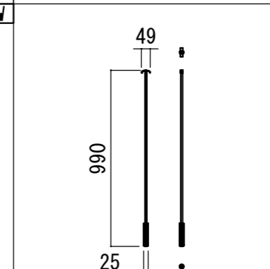
プルバー(引下げ棒) S=1:30
