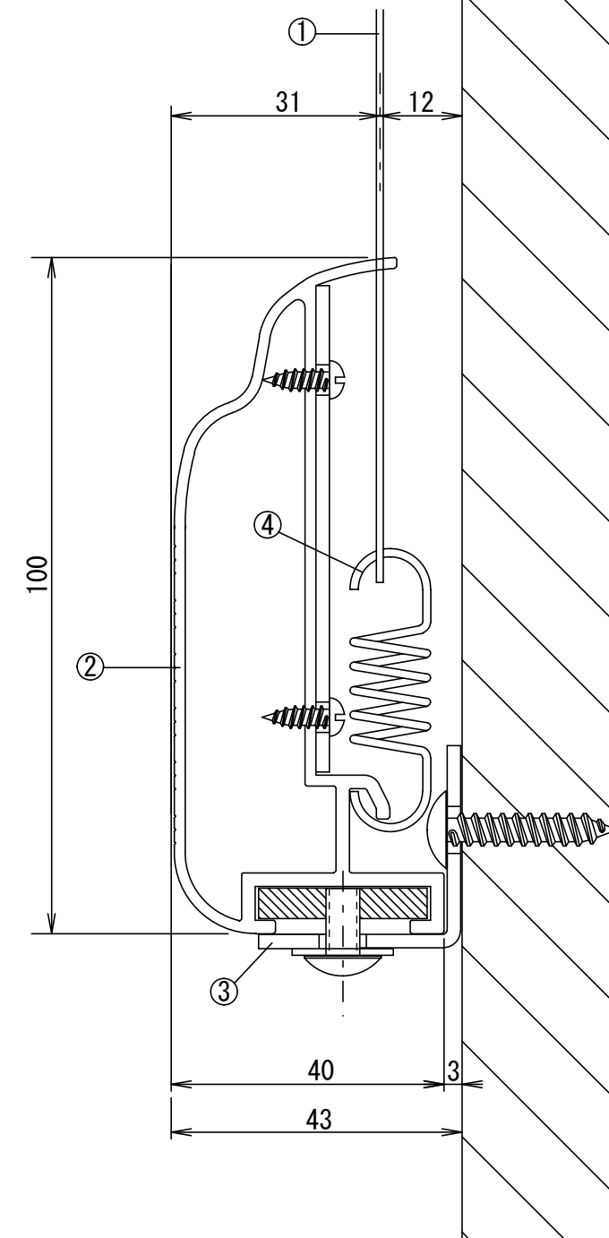
A 断面図 S = 1 / 1
