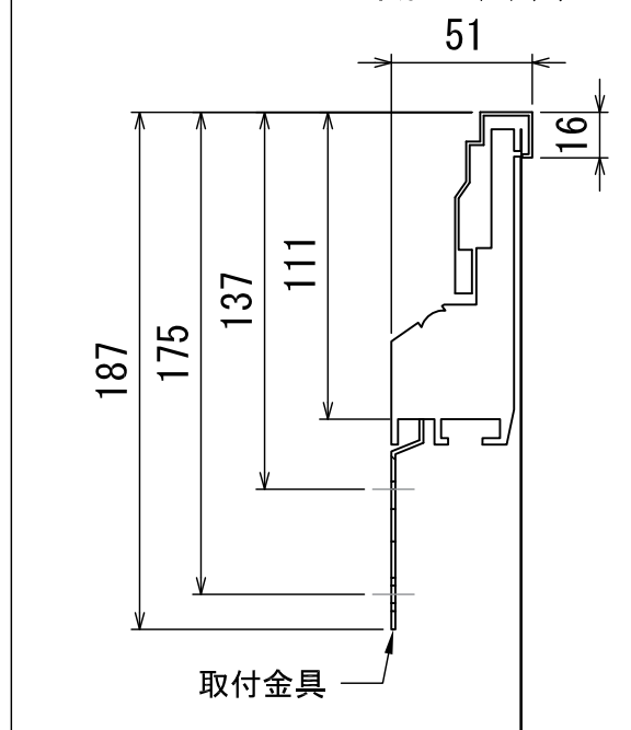
拡大図 S=1:3 外形寸法 (C)
