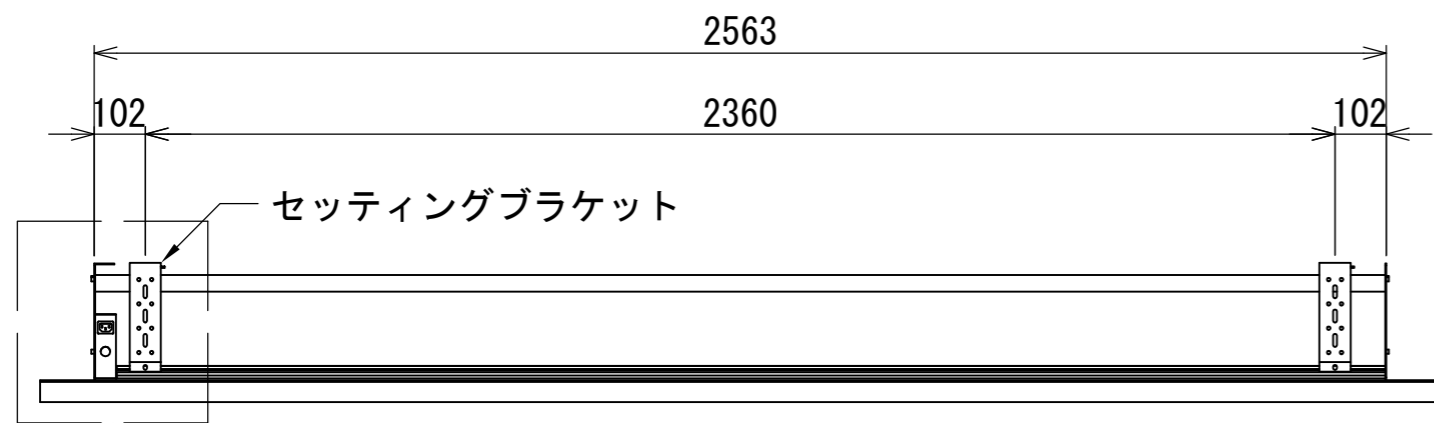
【詳細A】
