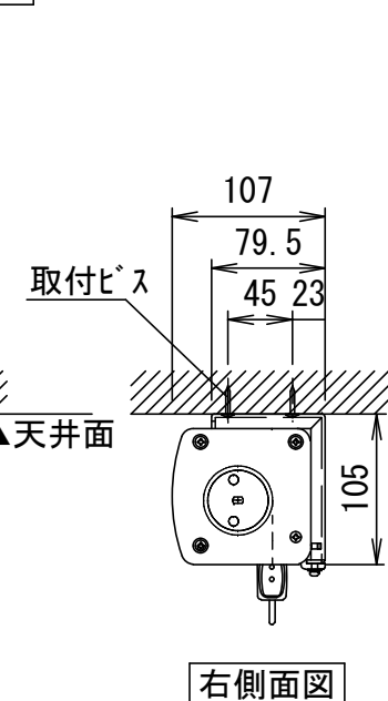
詳細図
