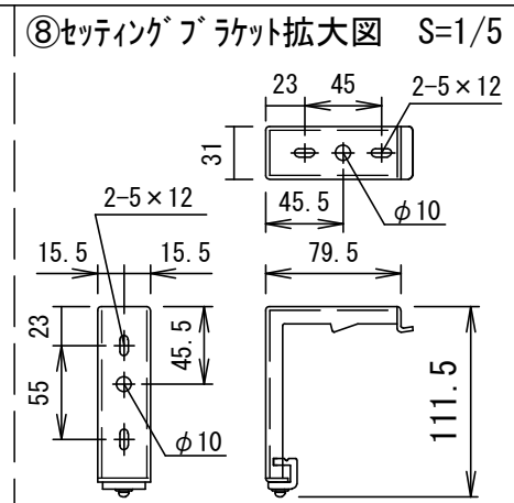
天井取付時
