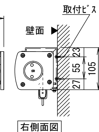
右側面図
