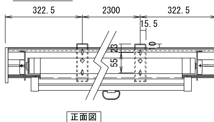
壁面取付時
