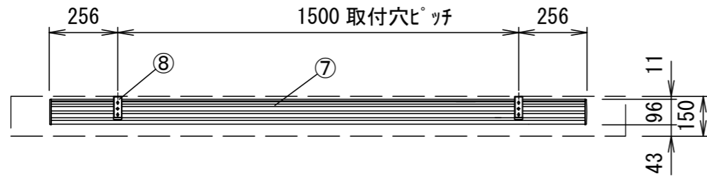
平面図
