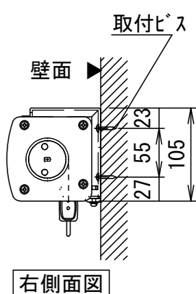
右側面図
