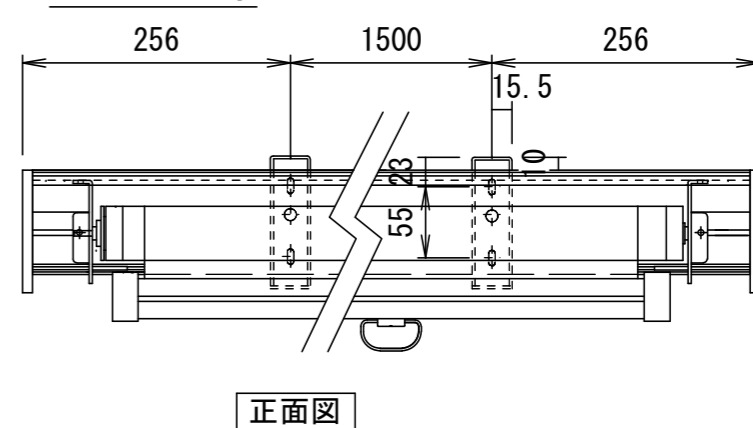
壁面取付時
