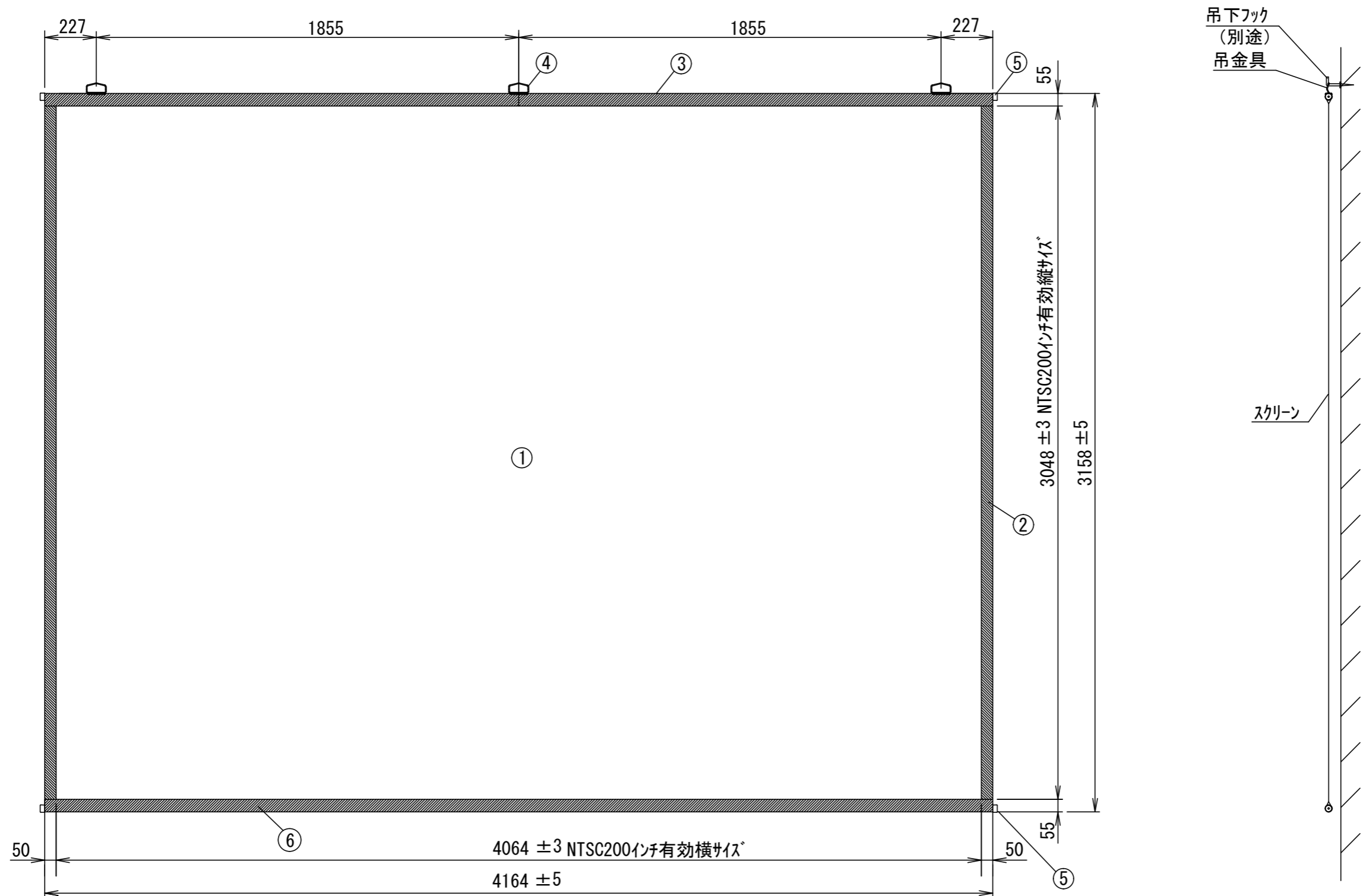
正面図
