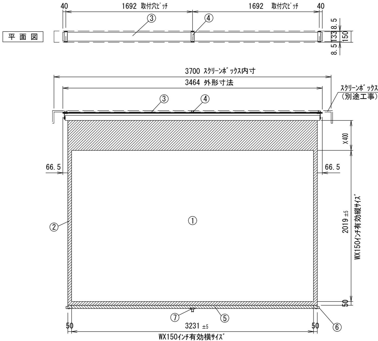
正面図
