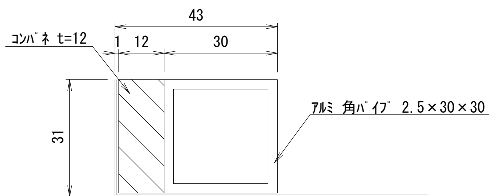
背面図
