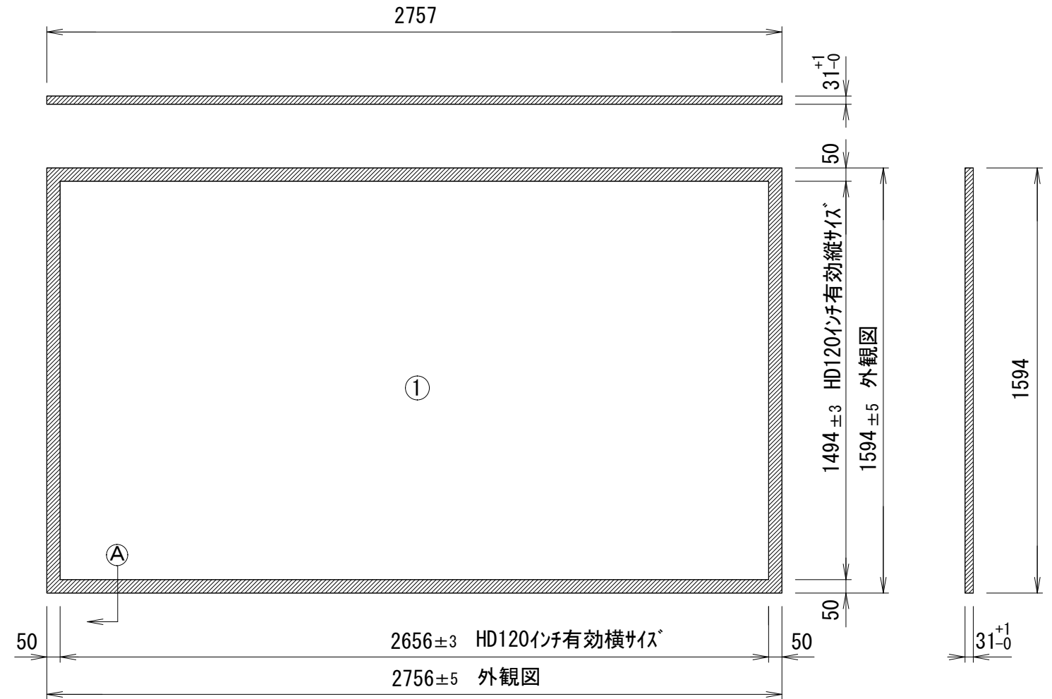
平面図
